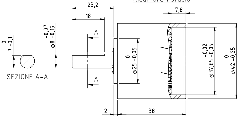
Riduttore 1 stadio
